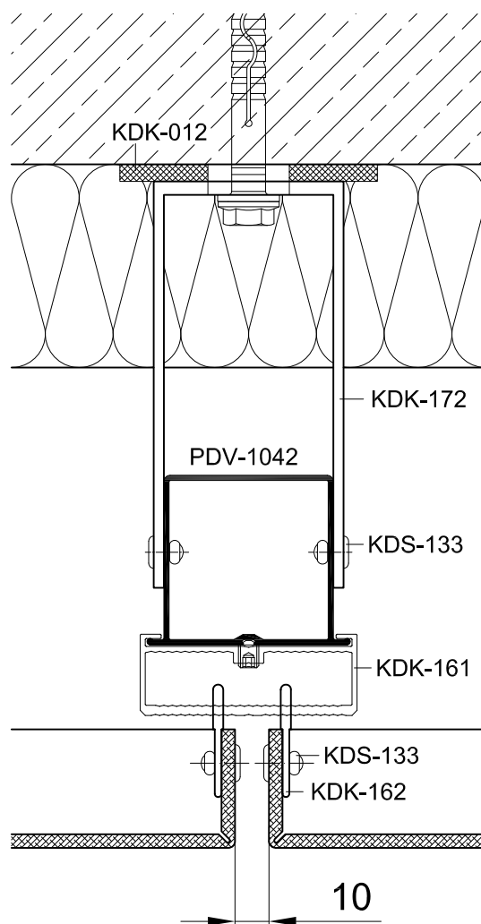
Кронштейны серии Ultra. Направляющая PDV-1042
